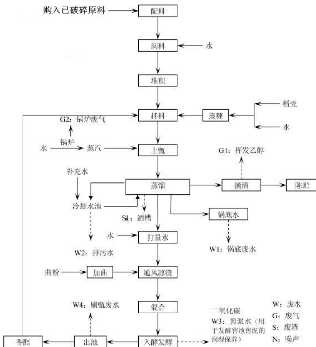
图 3.5-1 酿造生产流程及主要排污节点图
