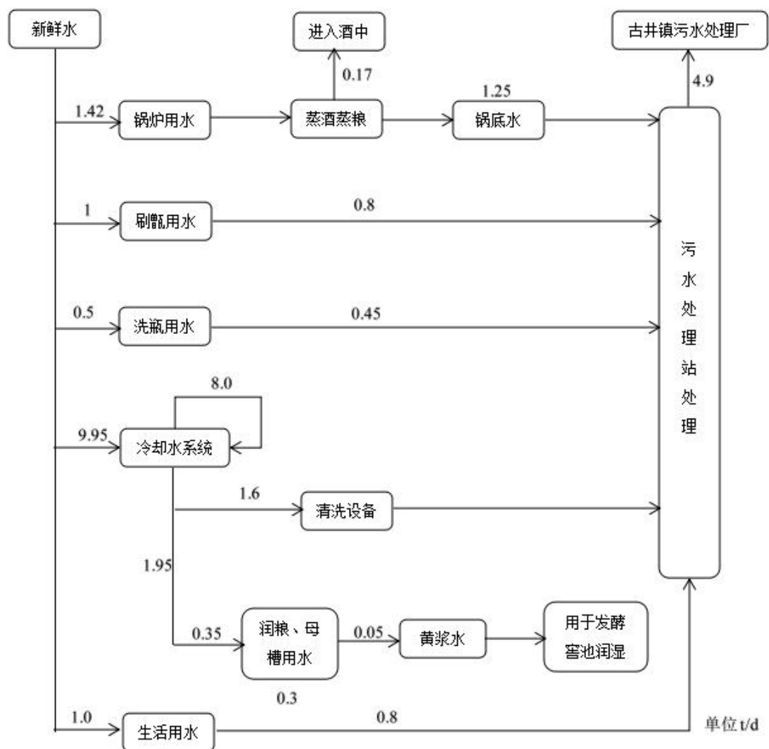
图 3.4-1 本项目水量平衡图 (m³/d)
