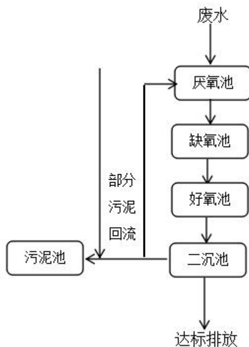
图 4.1-1 污水处理工艺流程图
