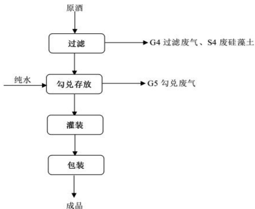
图 3.5-2 勾兑生产工艺流程图
