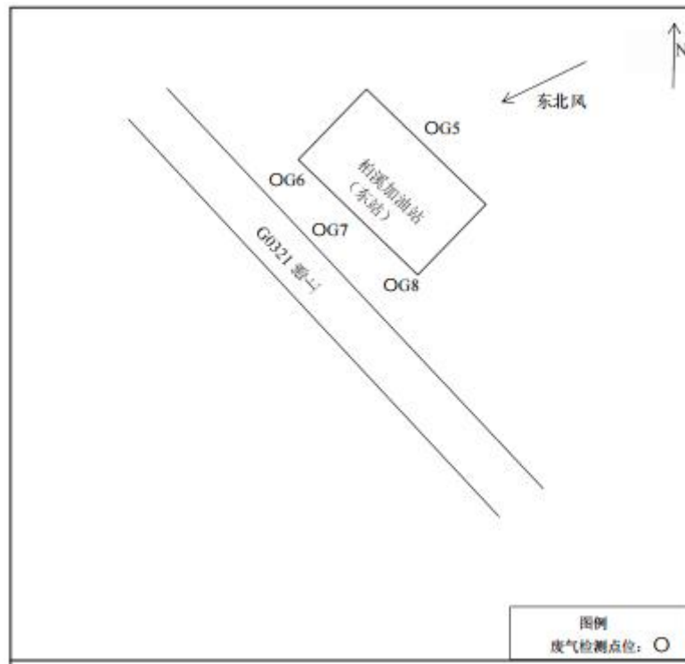
图 7-1 厂界无组织废气监测点位布置图
