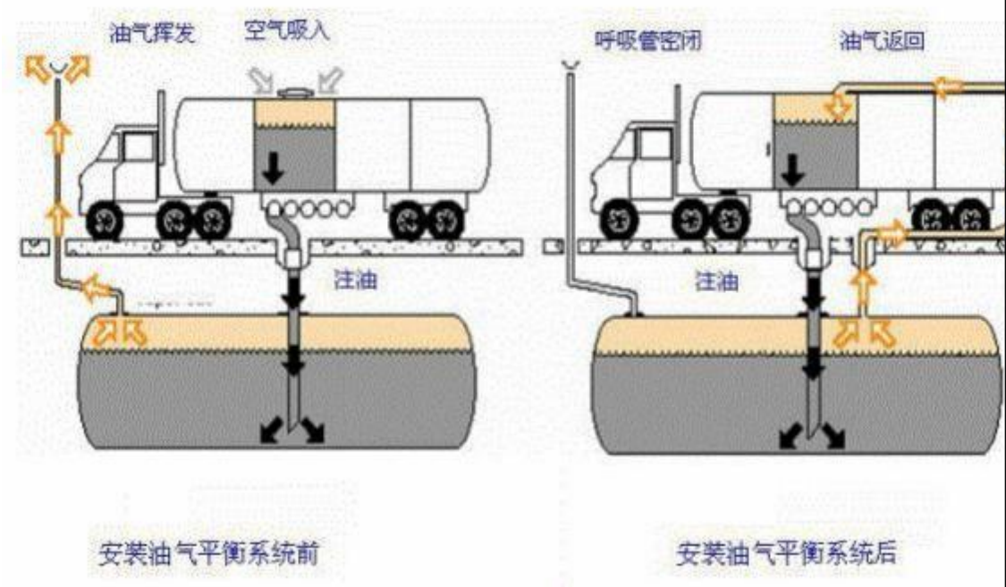
图 3-1 加油站卸油油气回收系统示意图
