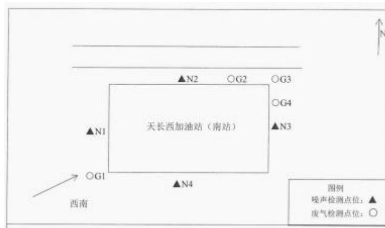
图 7-1 厂界无组织废气监测点位布置图
